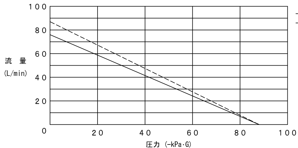
フィルター OF-2AL-TA (オプション品)
